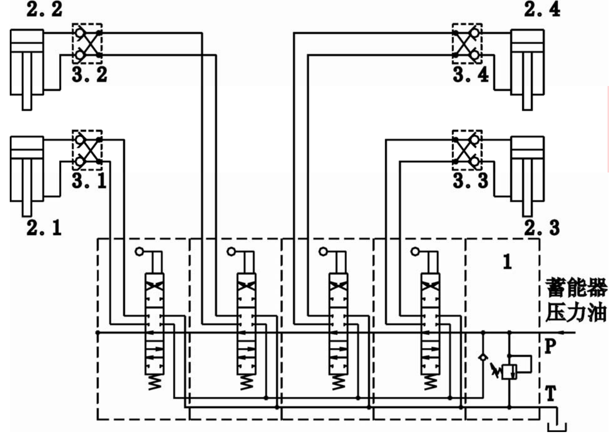
平衡阀工作原理图
