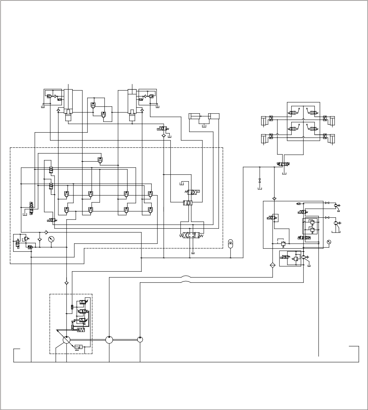
图7-1 主系统液压原理图
