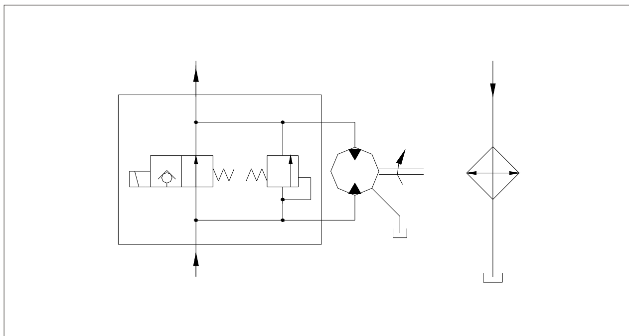
图7-3 风冷系统液压原理图
