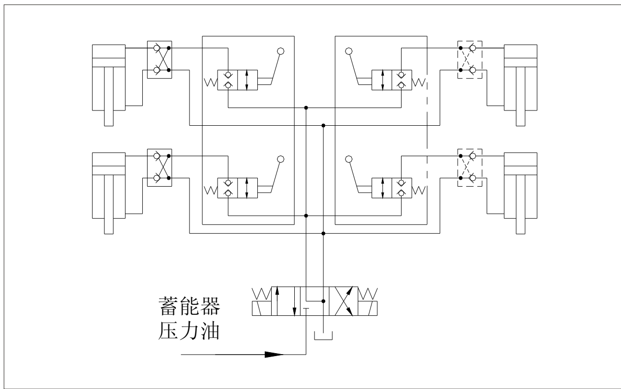
图7-2 支腿液压原理图
