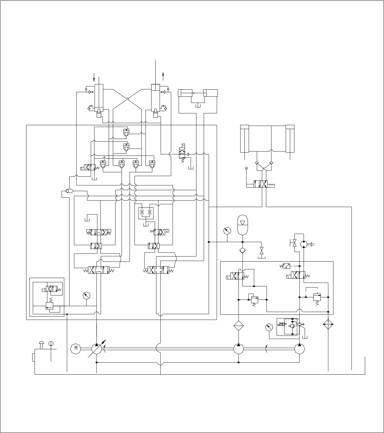
图7-1 液压原理图
