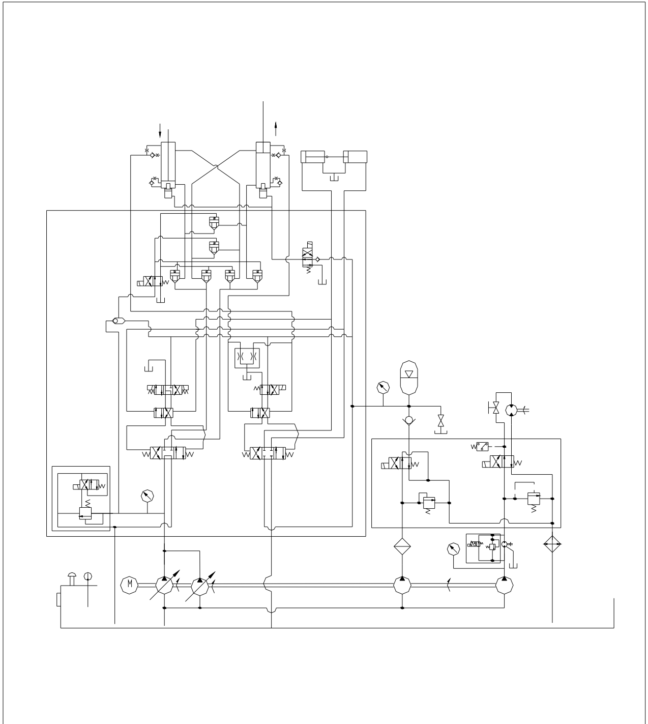
图7-1 液压原理图
