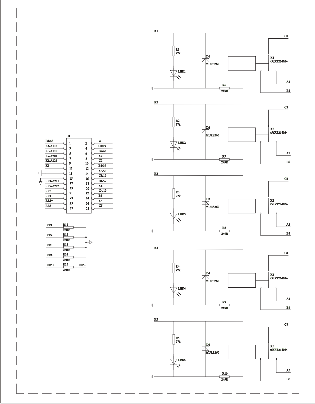
图7-13 继电器电路板
