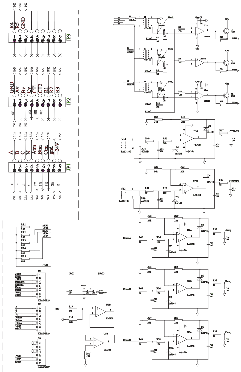
图7-14 三相采集电路板
