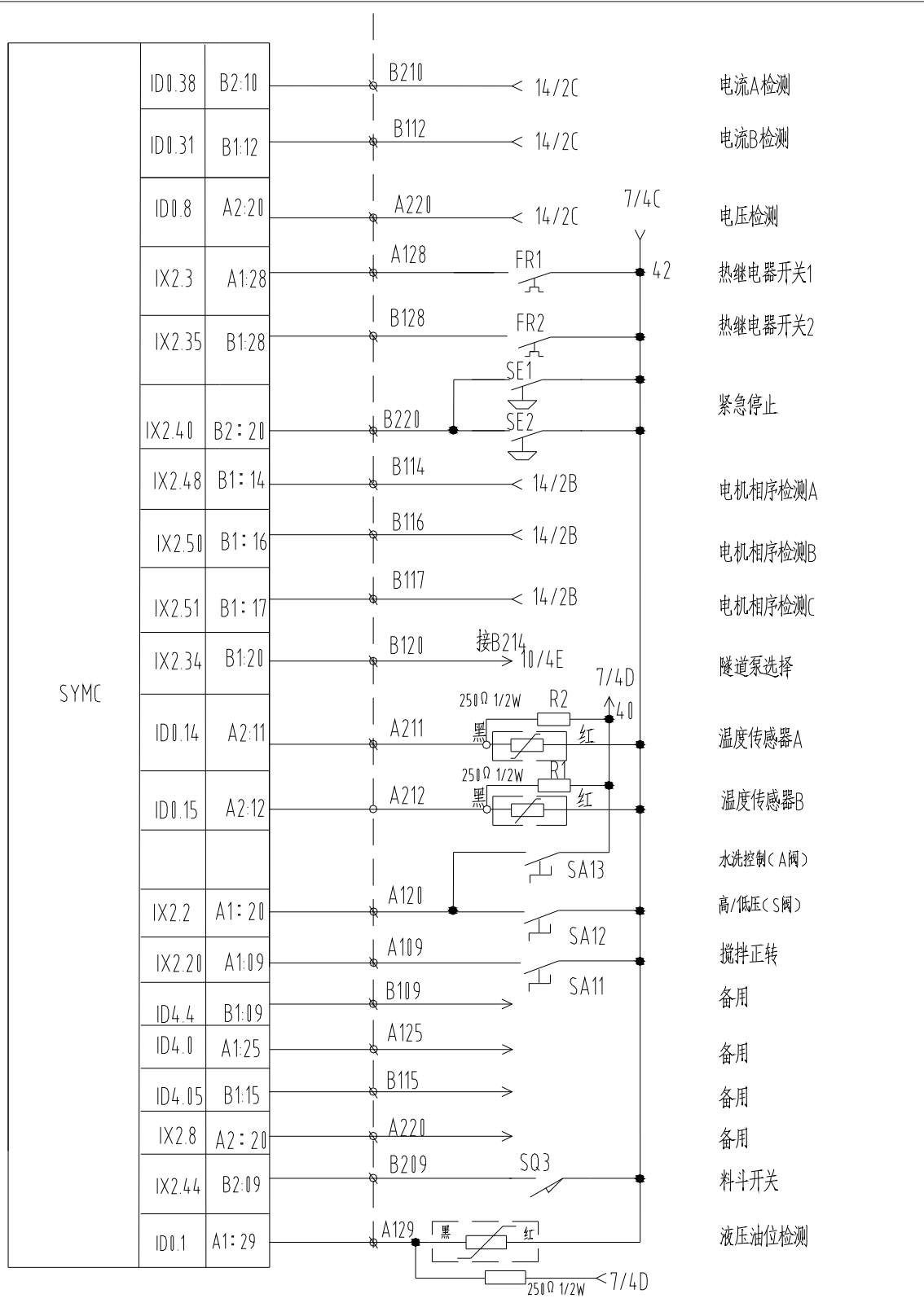
图7-10 输入回路2
