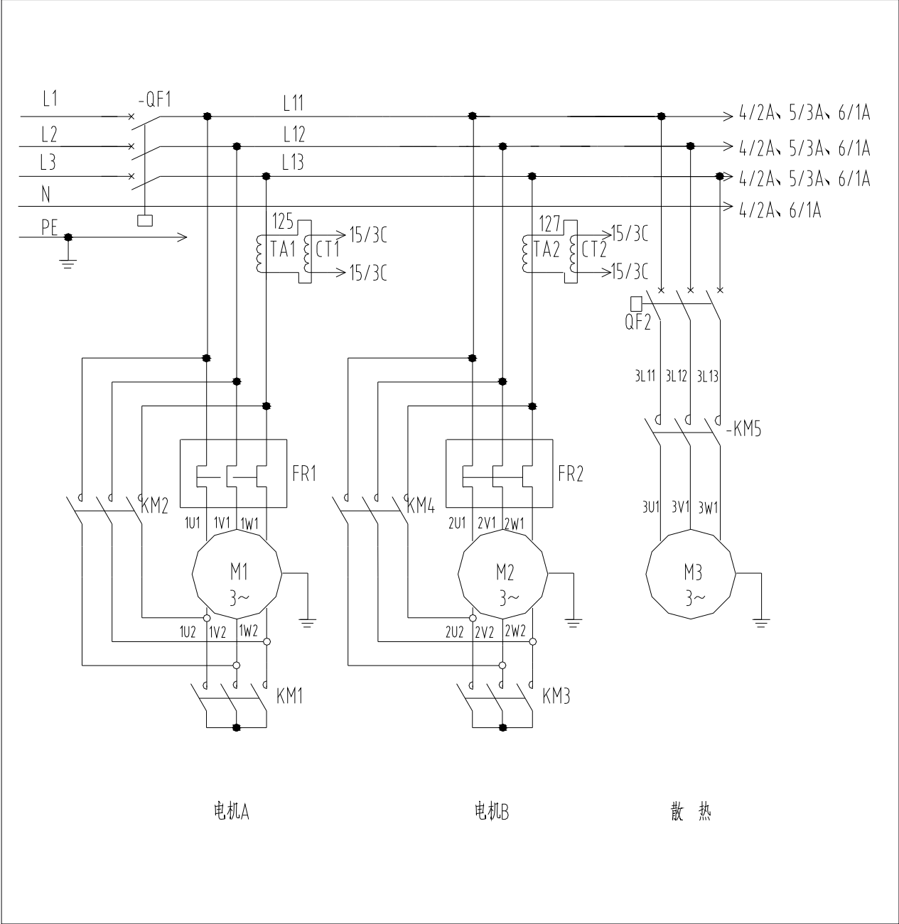
图7-2 主电路图
