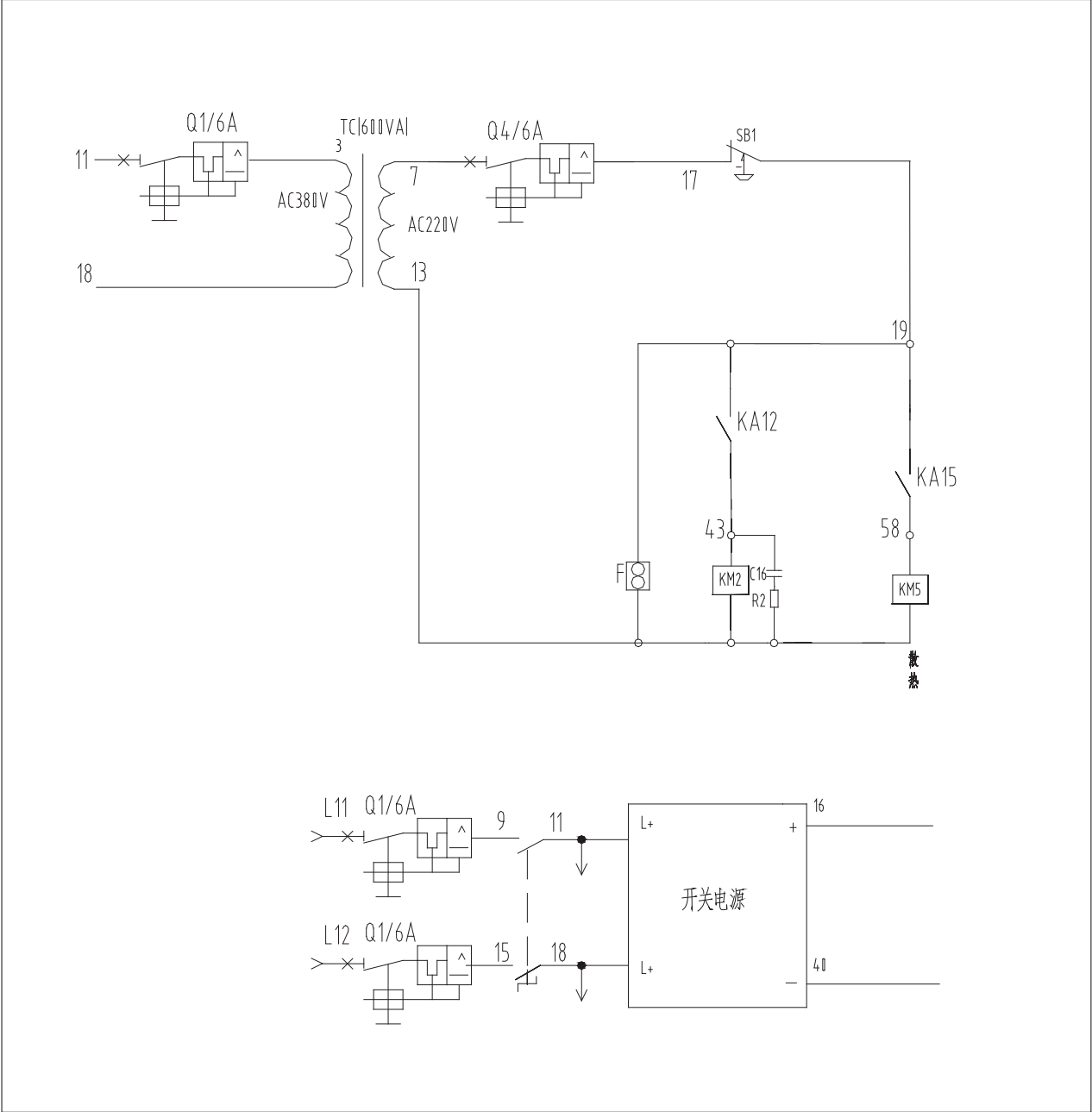
图7-3 软启动控制回路
