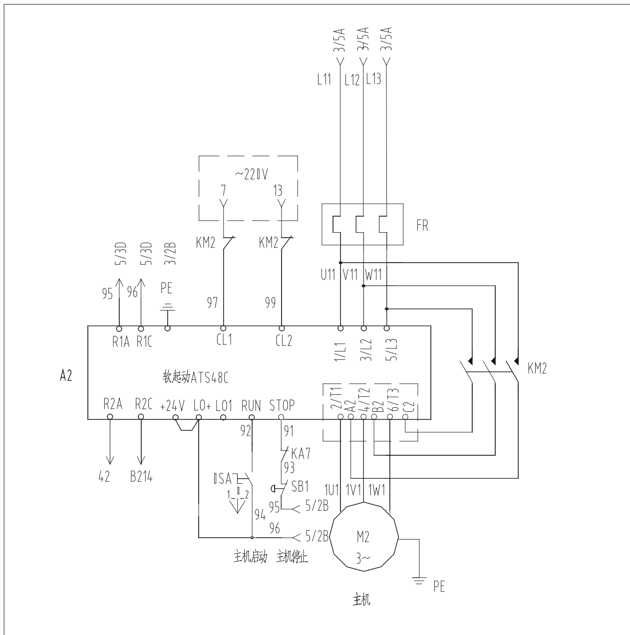
图7-4 软启动电路图
