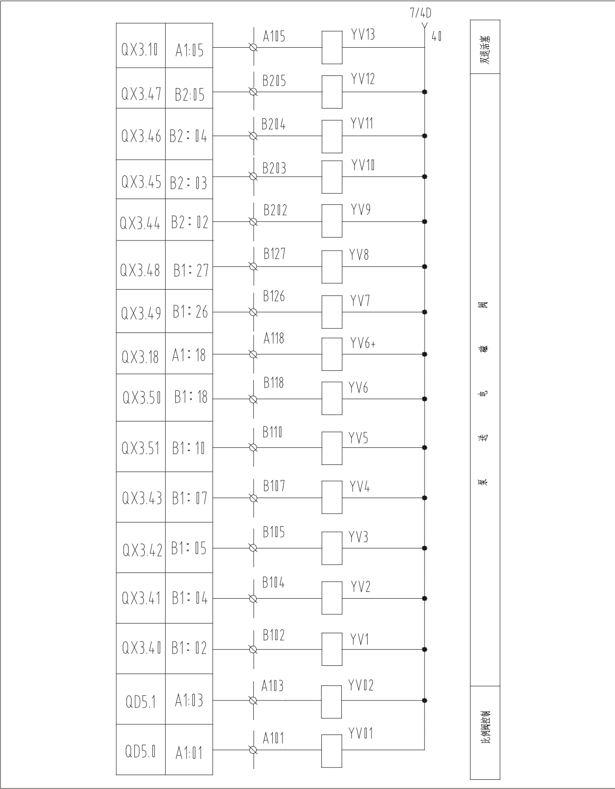
图7-7 电磁阀输出回路图
