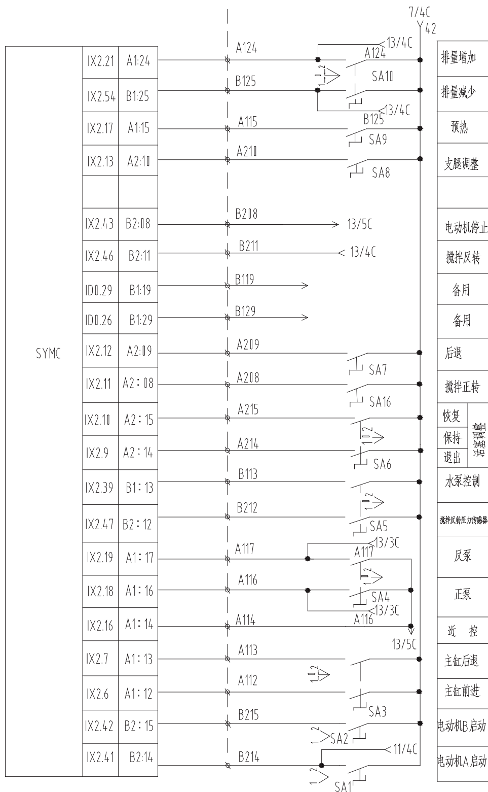
图7-9 输入回路1
