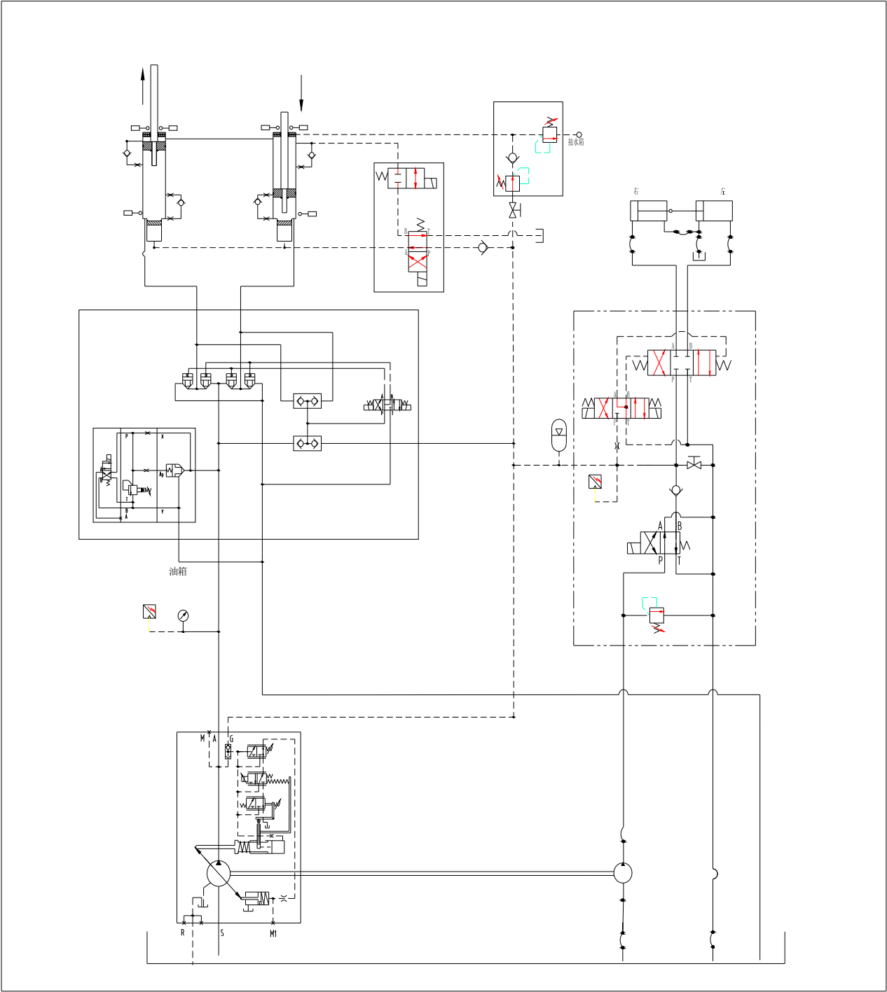
图7-1 泵送液压原理图
