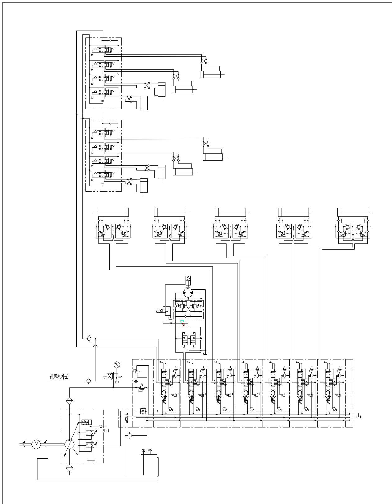
图7-2 臂架液压原理图 (五节臂)
