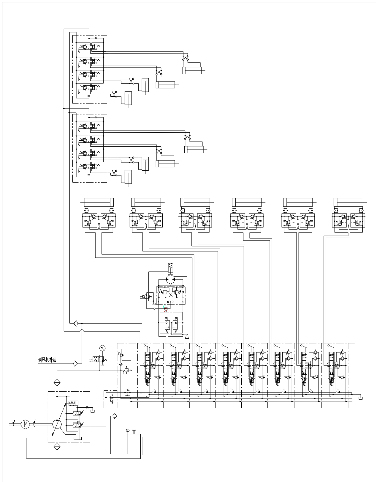
图7-3 臂架液压原理图(六节臂)
