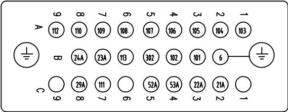
接收机输出接线端子线号示意图
