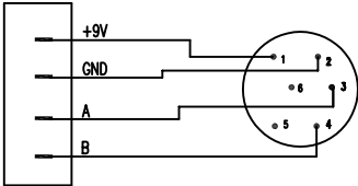
有线控制接线示意图
