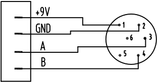
遥控有线控制接线示意图
